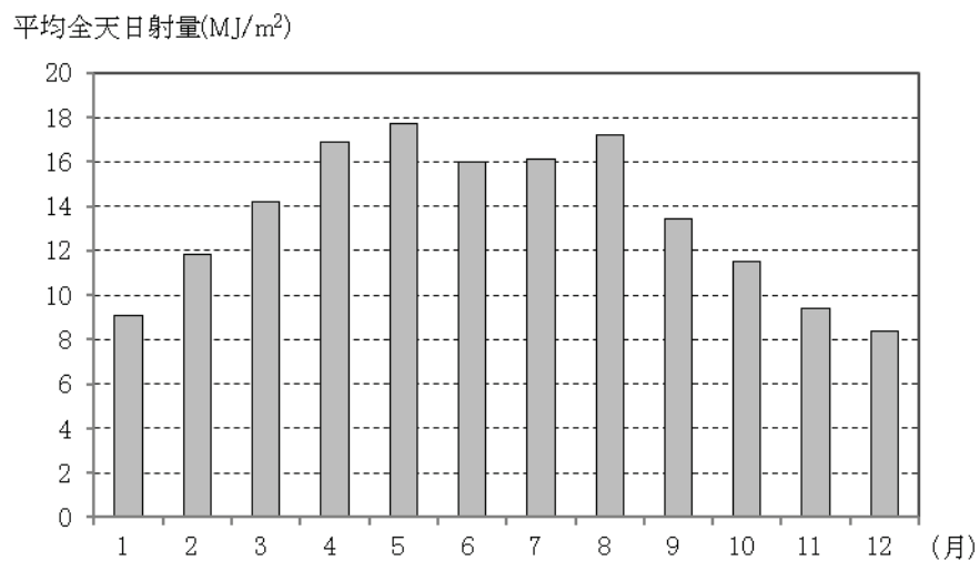
図 3.2.4 名古屋地方気象台における月別平均全天日射量の平年値 (統計期間 昭和56年(1981年)～平成22年(2010年))
