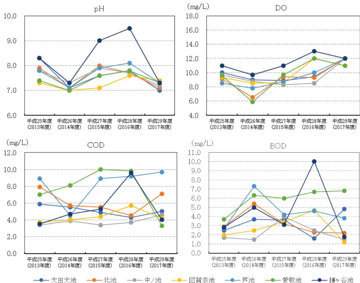
図 3.2.17 ため池の水質調査項目の経年変化
