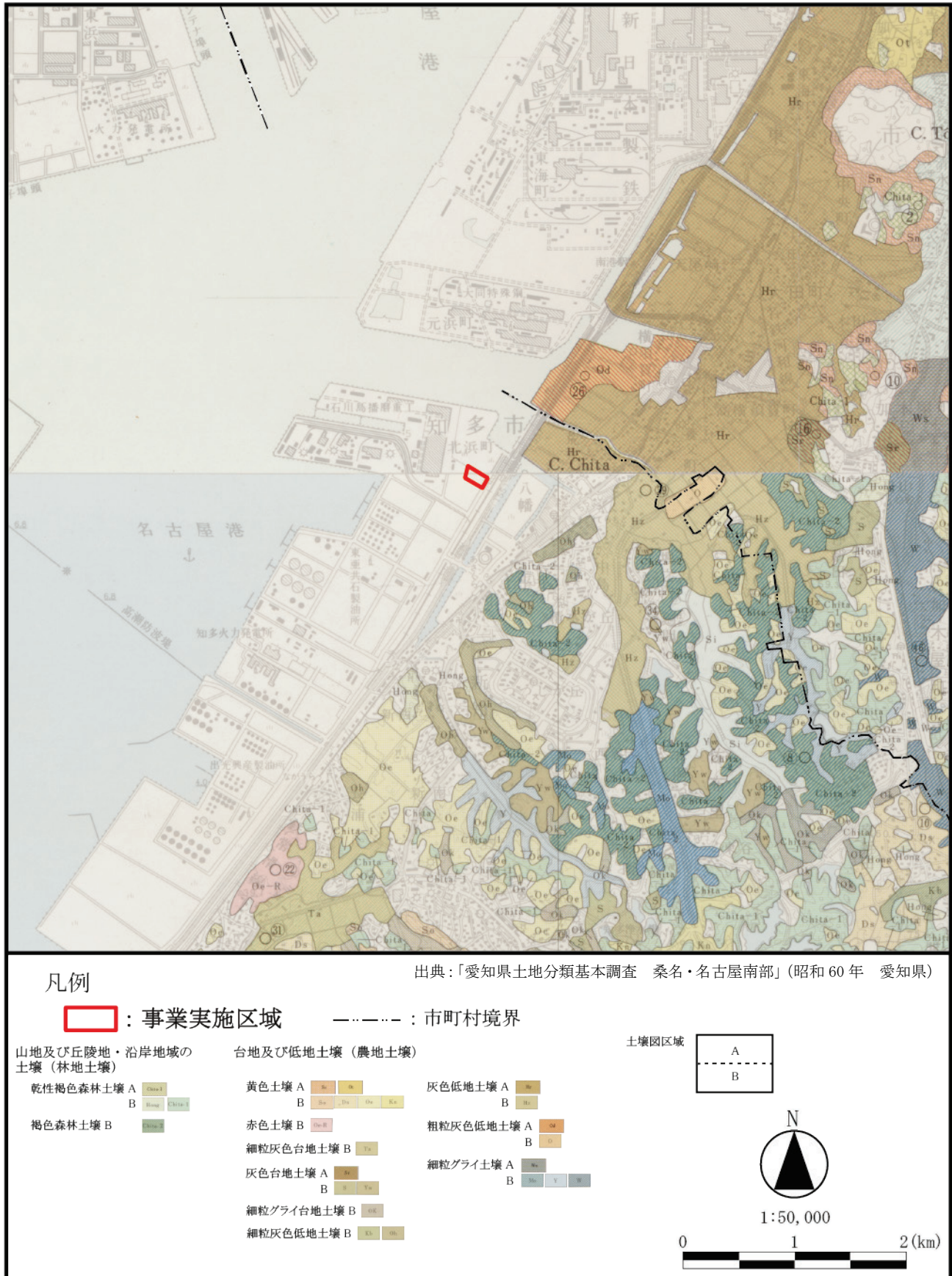
図 3.2.21 事業実施区域周辺における土壌の状況
