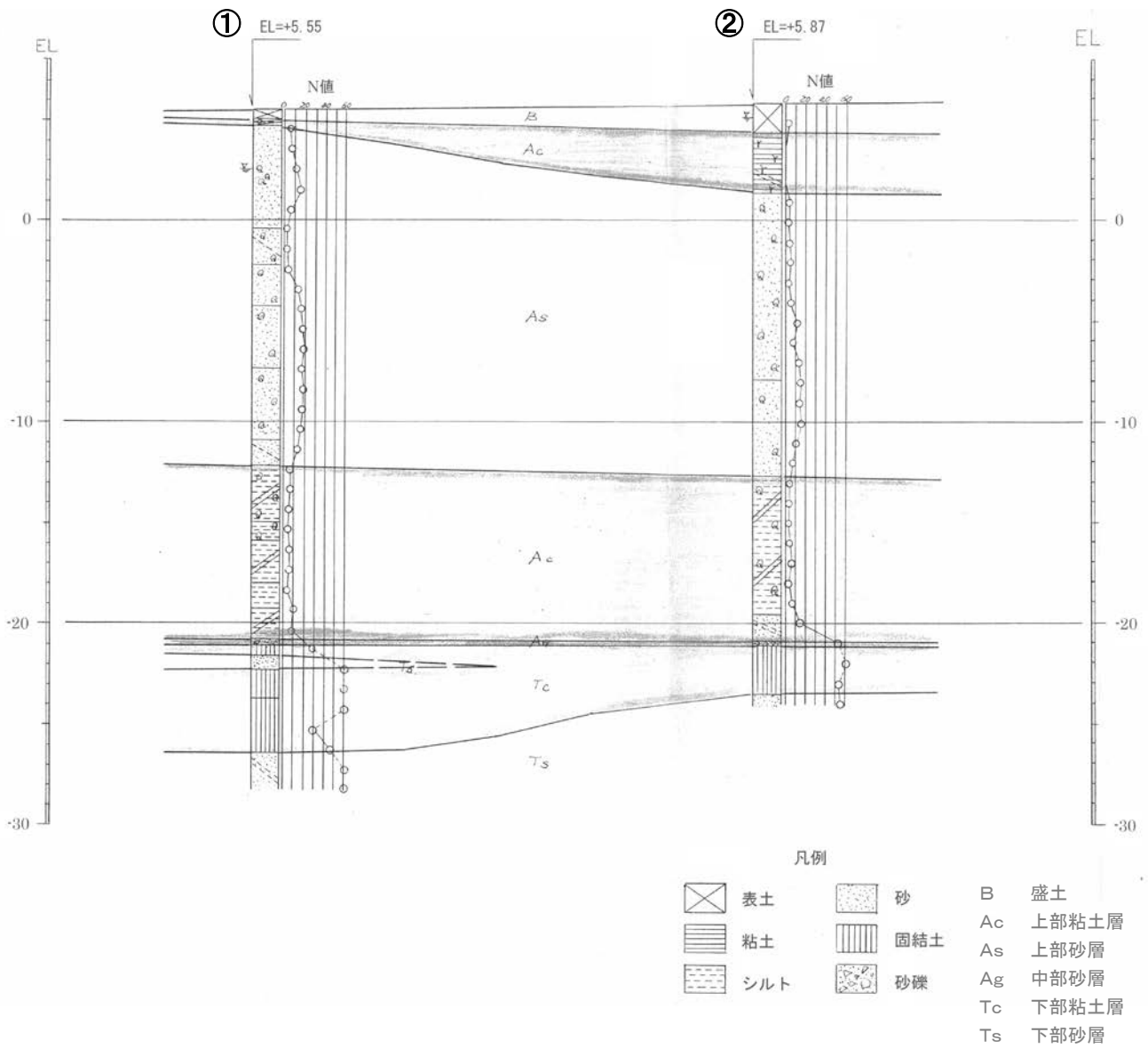
図 3.2.21 事業実施区域におけるボーリング調査結果
