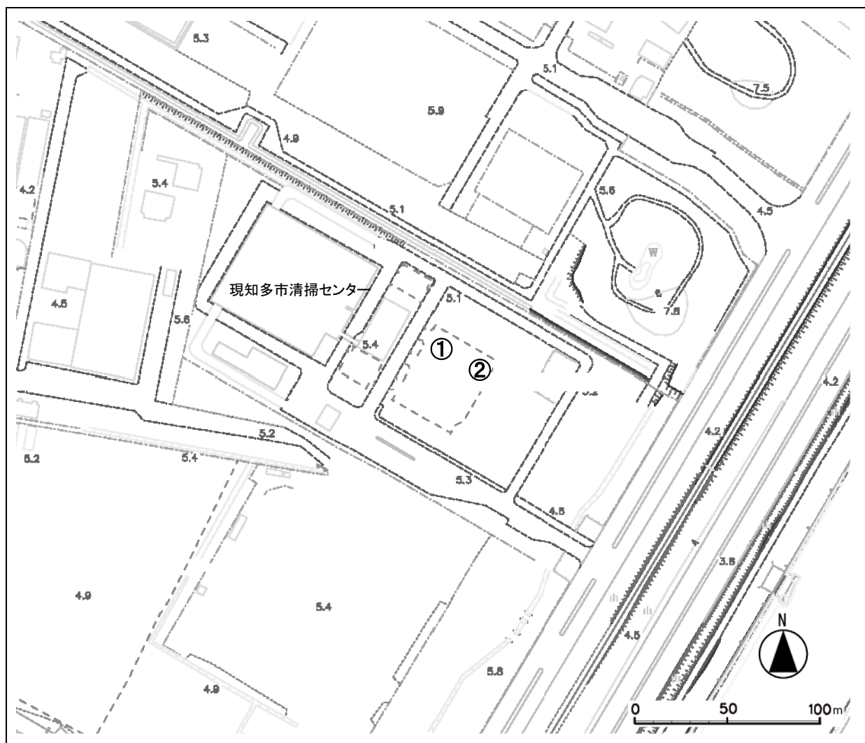
図 3.2.20 ボーリング調査地点
