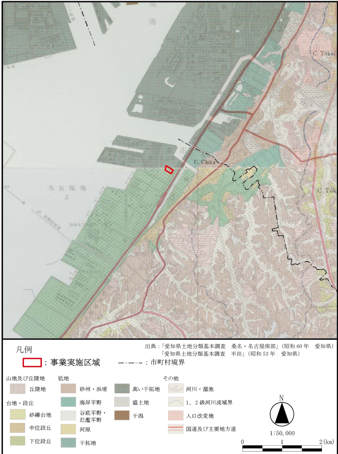
図 3.2.16 事業実施区域周辺における地形の状況
