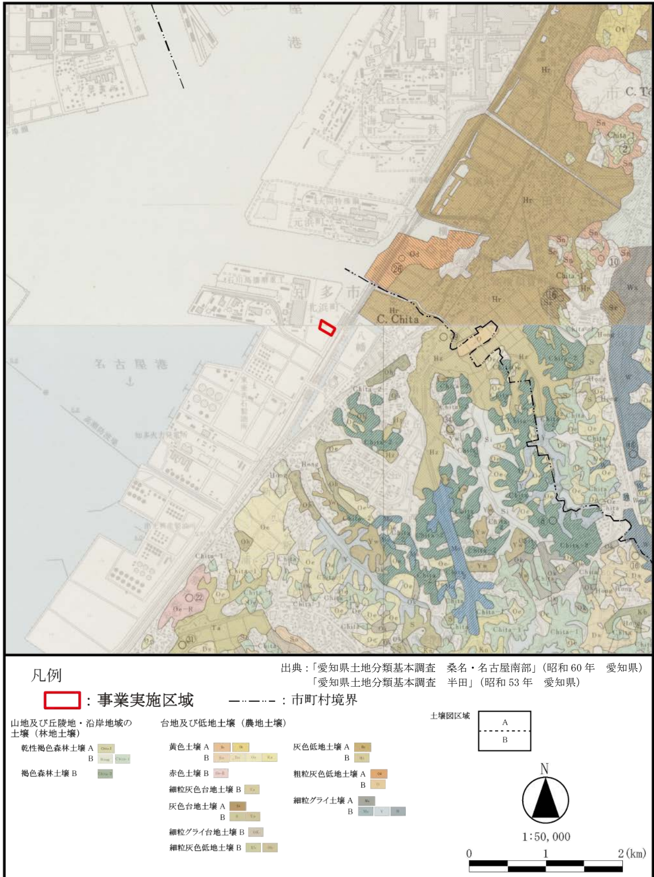
図 3.2.19 事業実施区域周辺における土壌の状況
