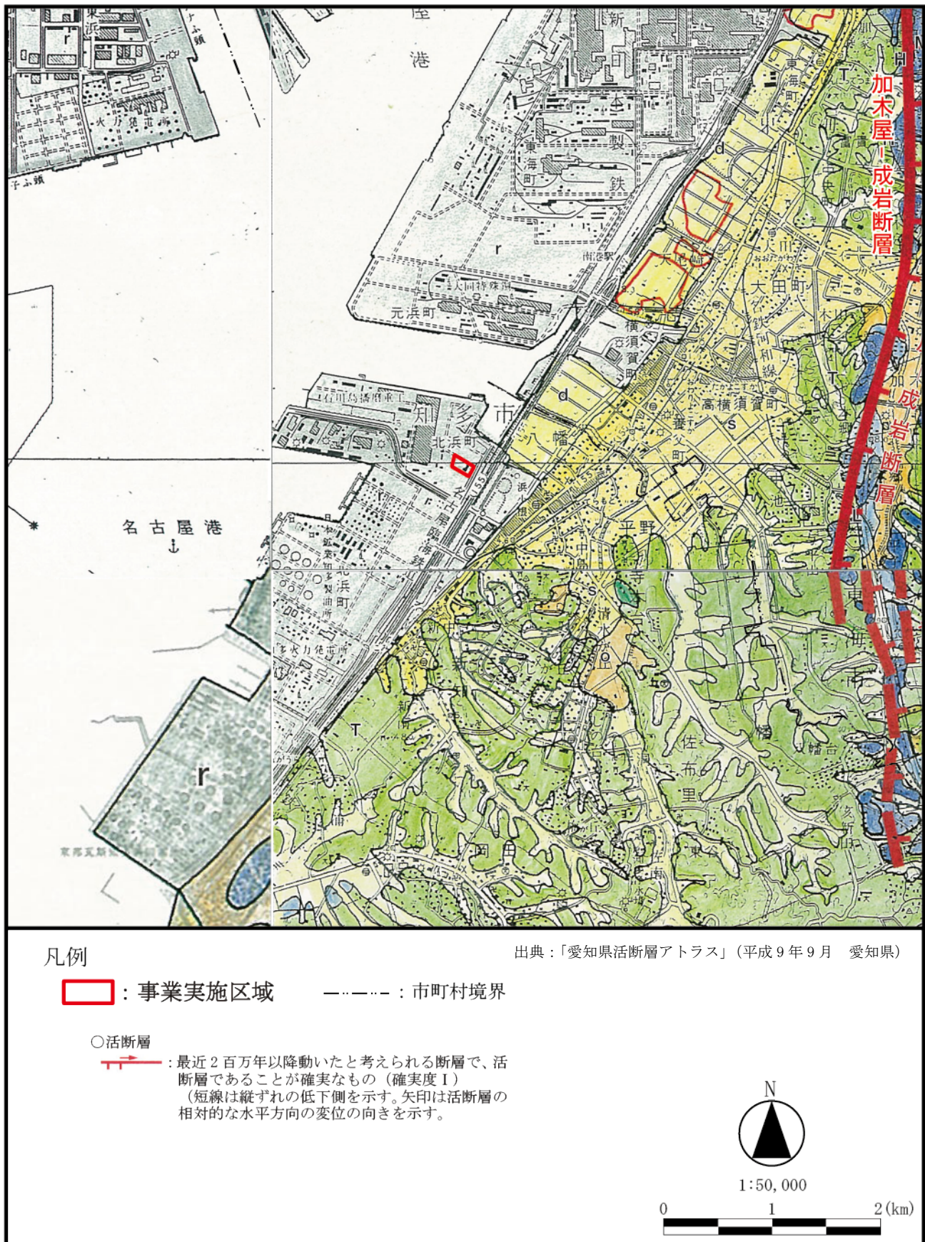
図 3.2.18 事業実施区域周辺における活断層の状況
