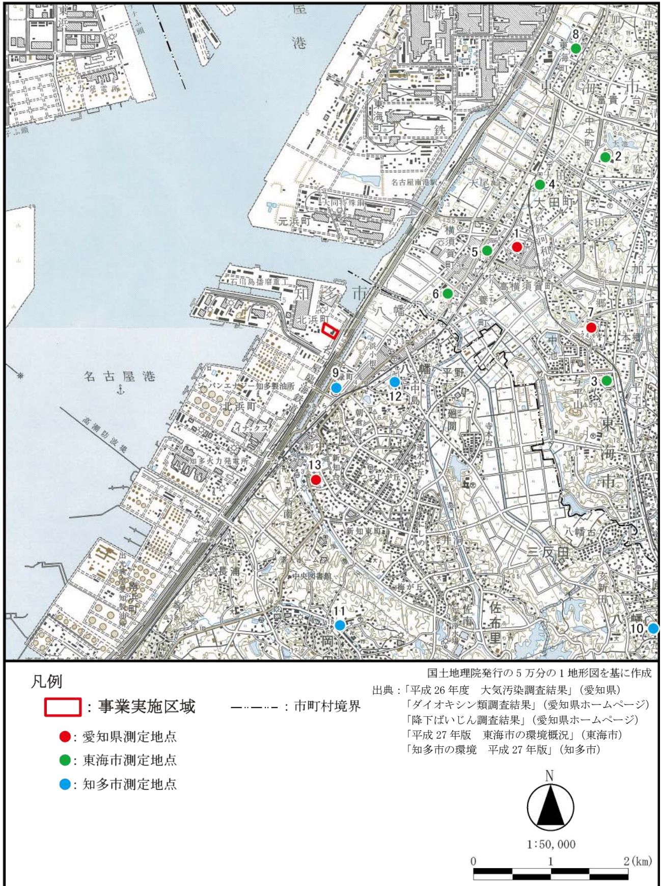
図 3.2.5 事業実施区域周辺における大気環境調査地点
