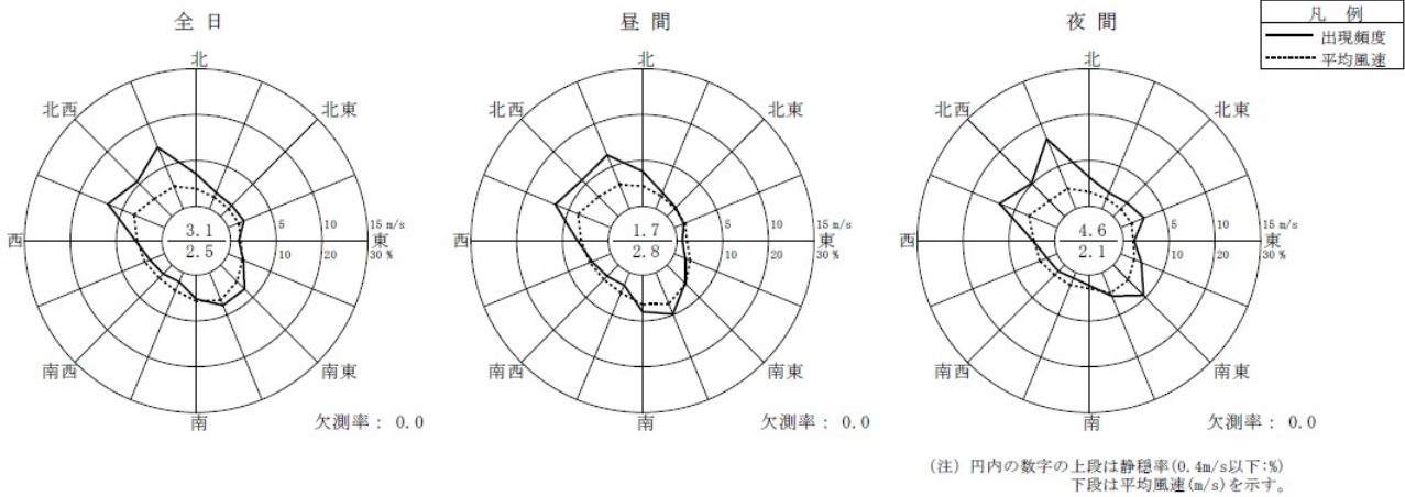
図 4.1.1 風配図（大府地域気象観測所）
