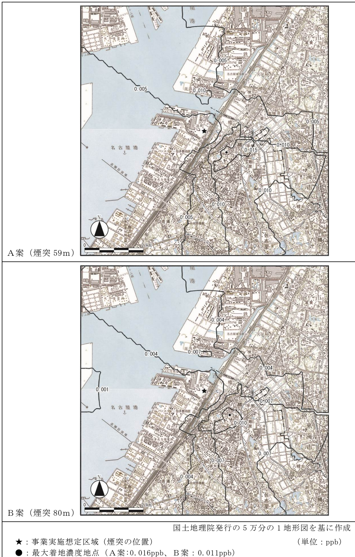
図 4.1.4 二酸化硫黄の予測結果（上段：A 案（59m）、下段：B 案（80m））
