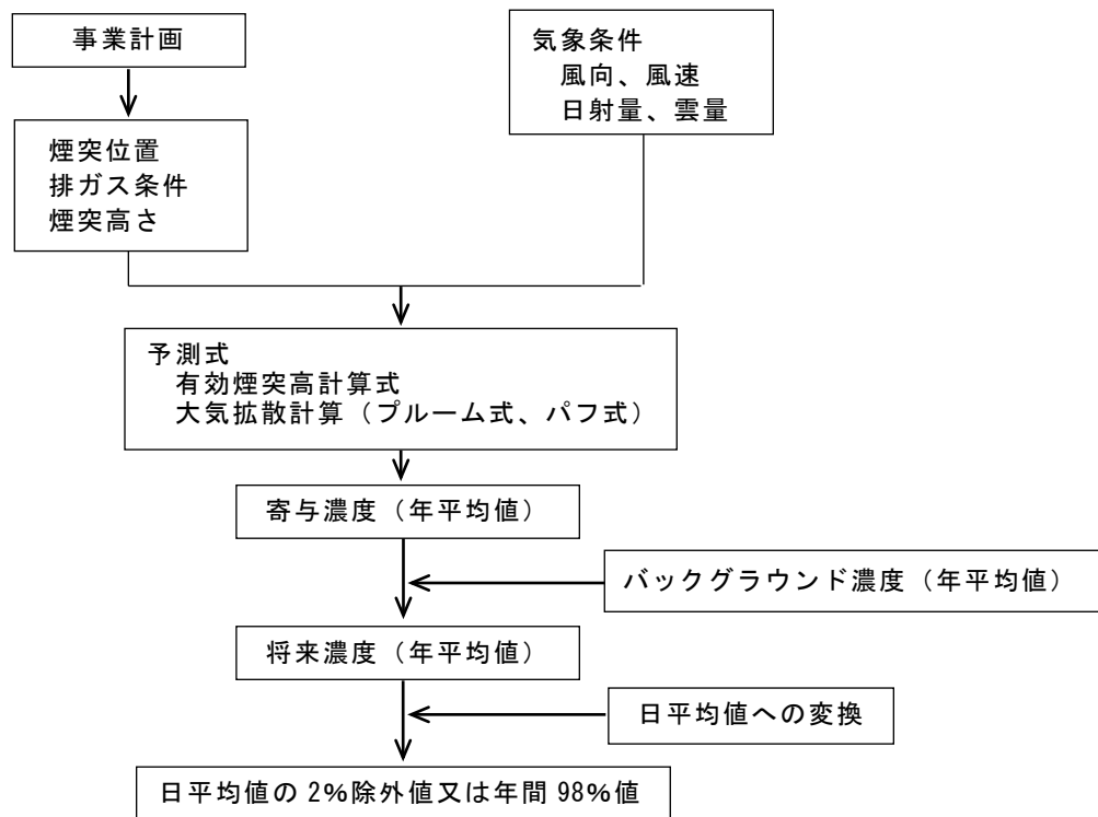
図 4.1.2 大気質の予測手順
