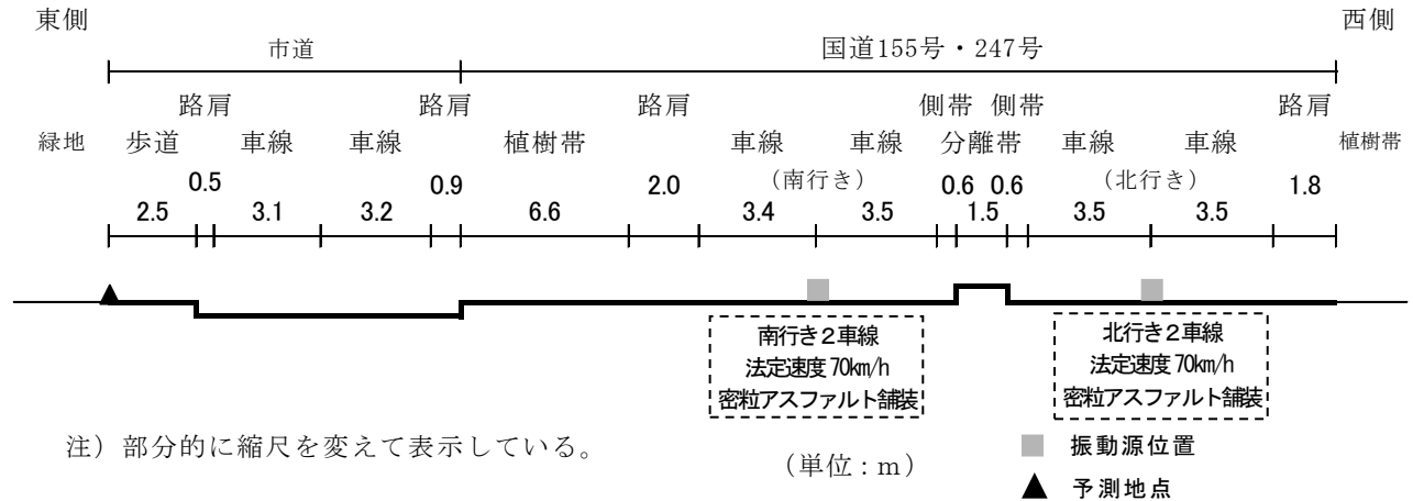
図 8.4.2 道路交通振動の予測地点の道路構造断面
